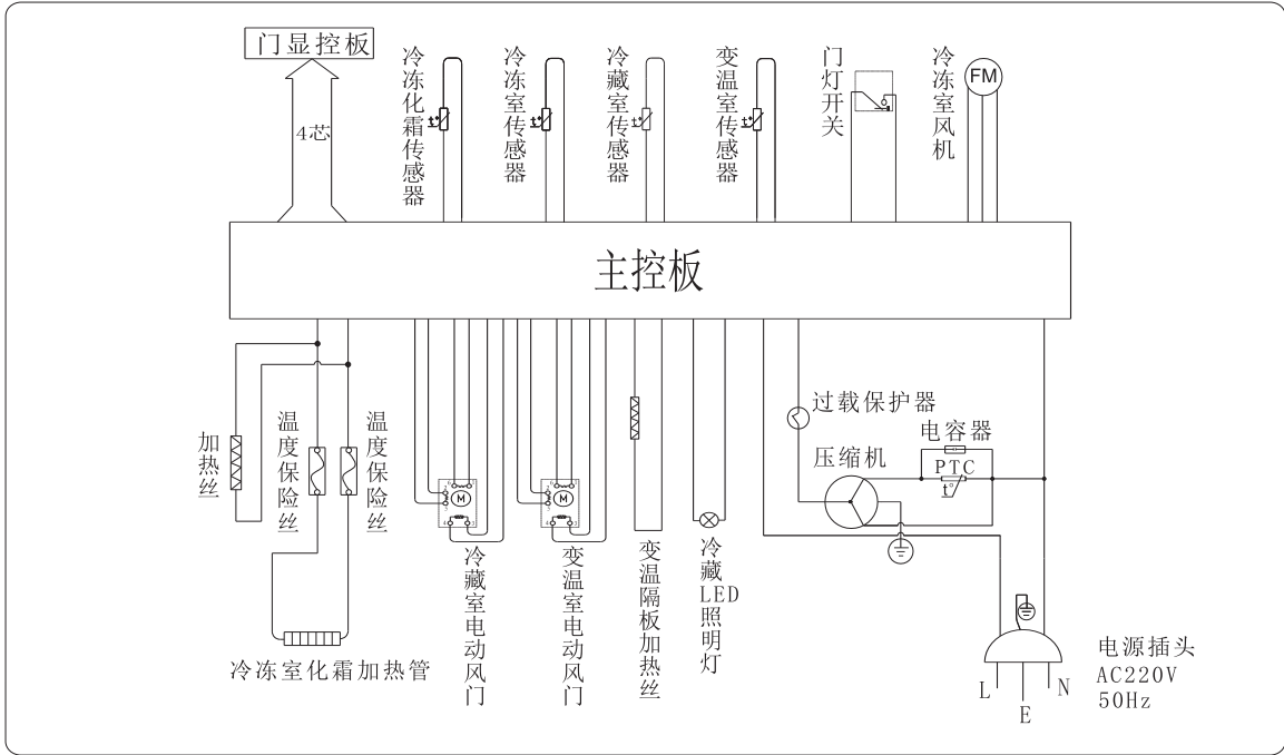
电路图（BCD-263WTGEW/BCD-263WT07GWS/BCD-262WT07DG）
