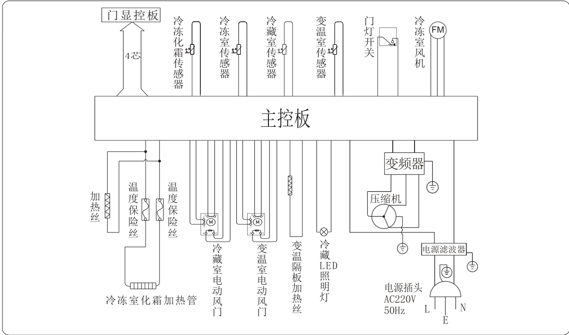
电路图（BCD-263WT07GBWS）
